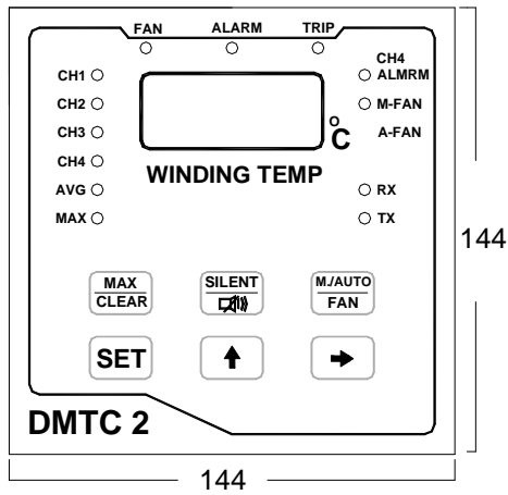
正視圖
