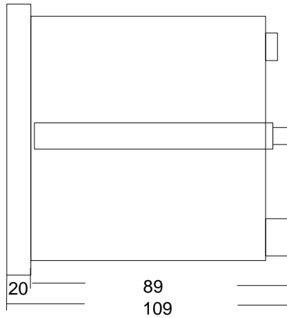
側視圖
