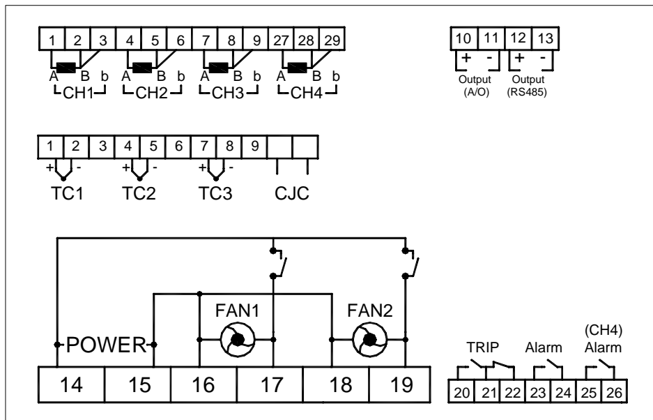
接線圖
