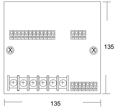
後視圖(開孔尺寸)
